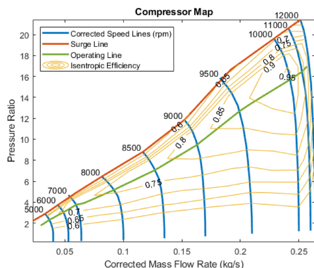
Fig. 27 TEMS compressor map
