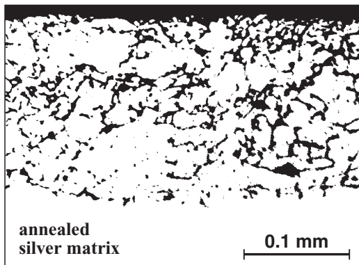
Metallograph (Bennett 1994)
